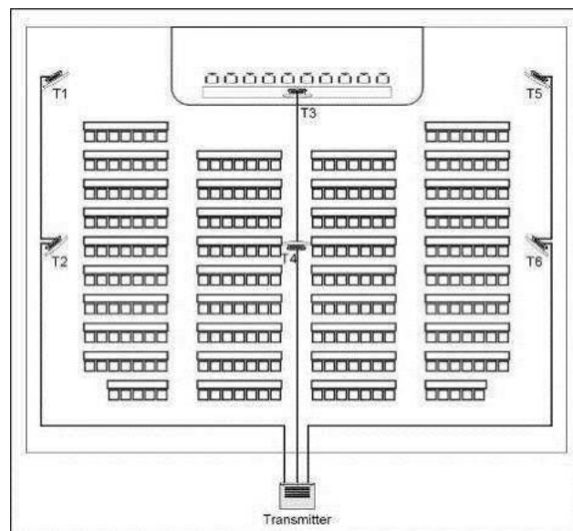
Рис. 3.8 Симметричное распределение кабелей в помещении
