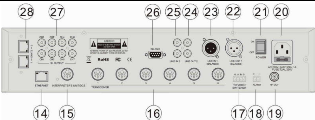
Задняя панель центрального блока HCS-5300MA/80
