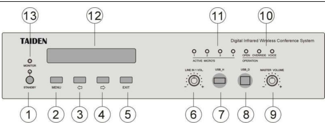
Передняя панель центрального блока HCS-5300M/80
