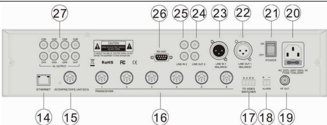
Задняя панель центрального блока HCS-5300MB/80
