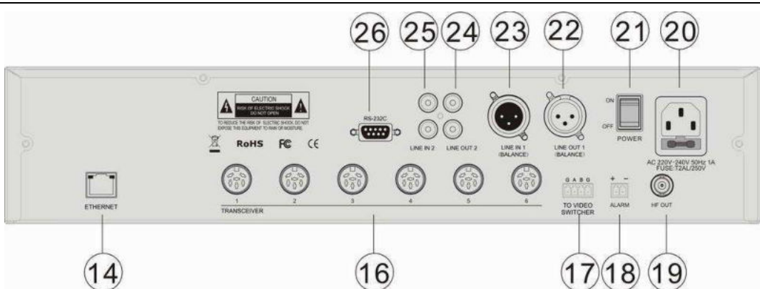
Задняя панель центрального блока HCS-5300MC/80
