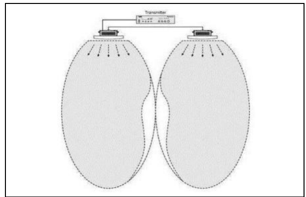
Рис. 1.14 Уменьшение зоны охвата вследствие разницы задержки в кабелях
