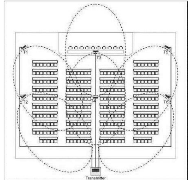
Рис. 1.11 Размещение ИК излучателей в конференц-зале с подиумом
